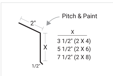
Eave (Style A Fascia)
